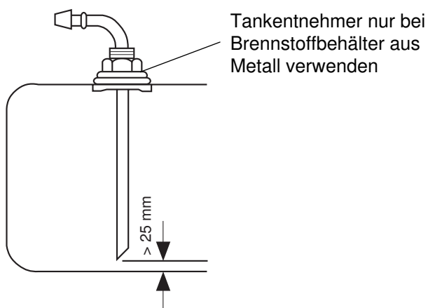
Abb. 805 Webasto-Tankentnehmer
